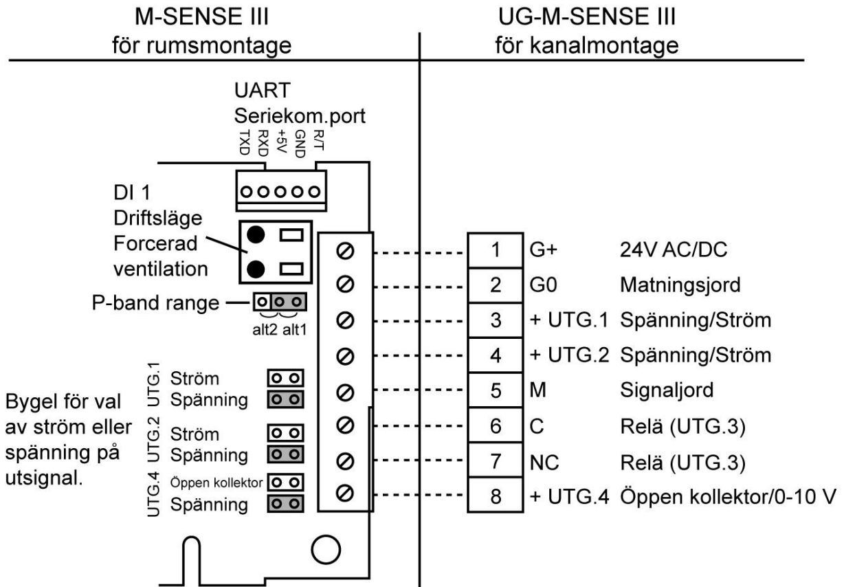
Anslutning av UG-M-SENSE III via skruvplinten vid kanalmontage.
