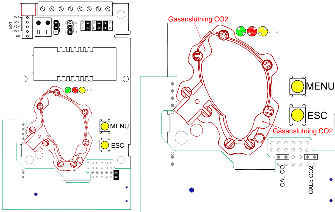
Kretskortet med kalibreringsbygeln i normalläge. En förstordad del av kretskortet med markerade gasanslutningar och bygellägen för kalibrering ses till höger.
